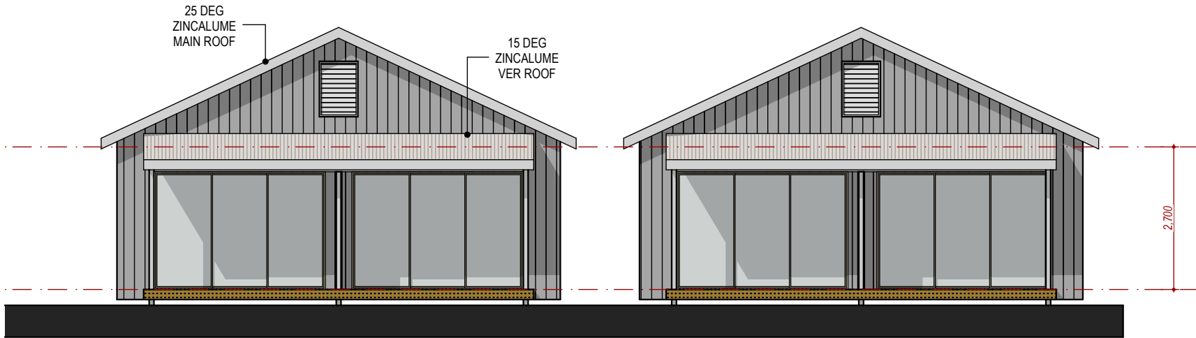
E1 FRONT ELEVATION 1:100
