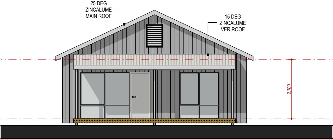
E1 FRONT ELEVATION 1:100
